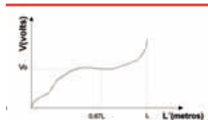
Figura 3. Curva de Potencial vs. Distancia
